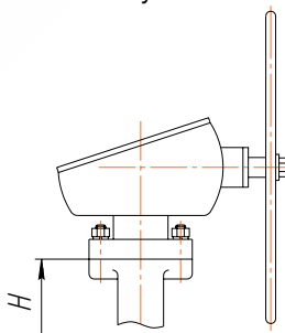
Рисунок 2. Исполнение с редуктором
