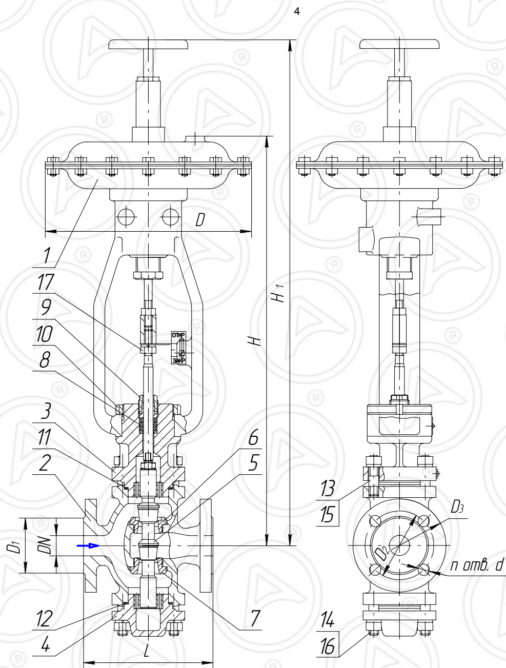
Рисунок 1 Основные узлы и габариты клапана НО
