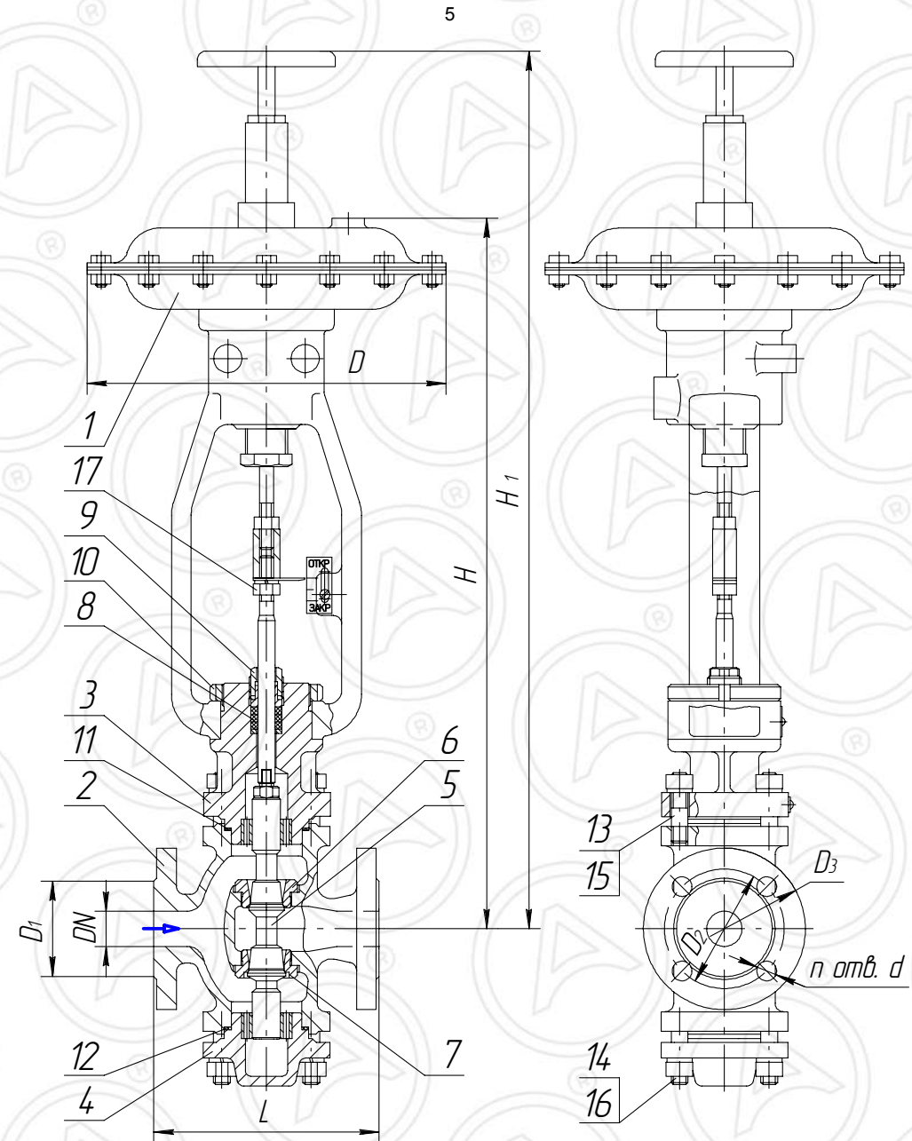
Рисунок 2 Основные узлы и габариты клапана НЗ
