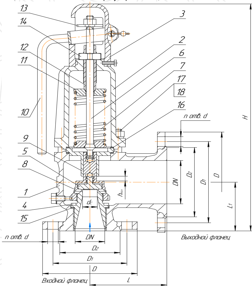
Рисунок 1. Основные узлы и габариты клапана
