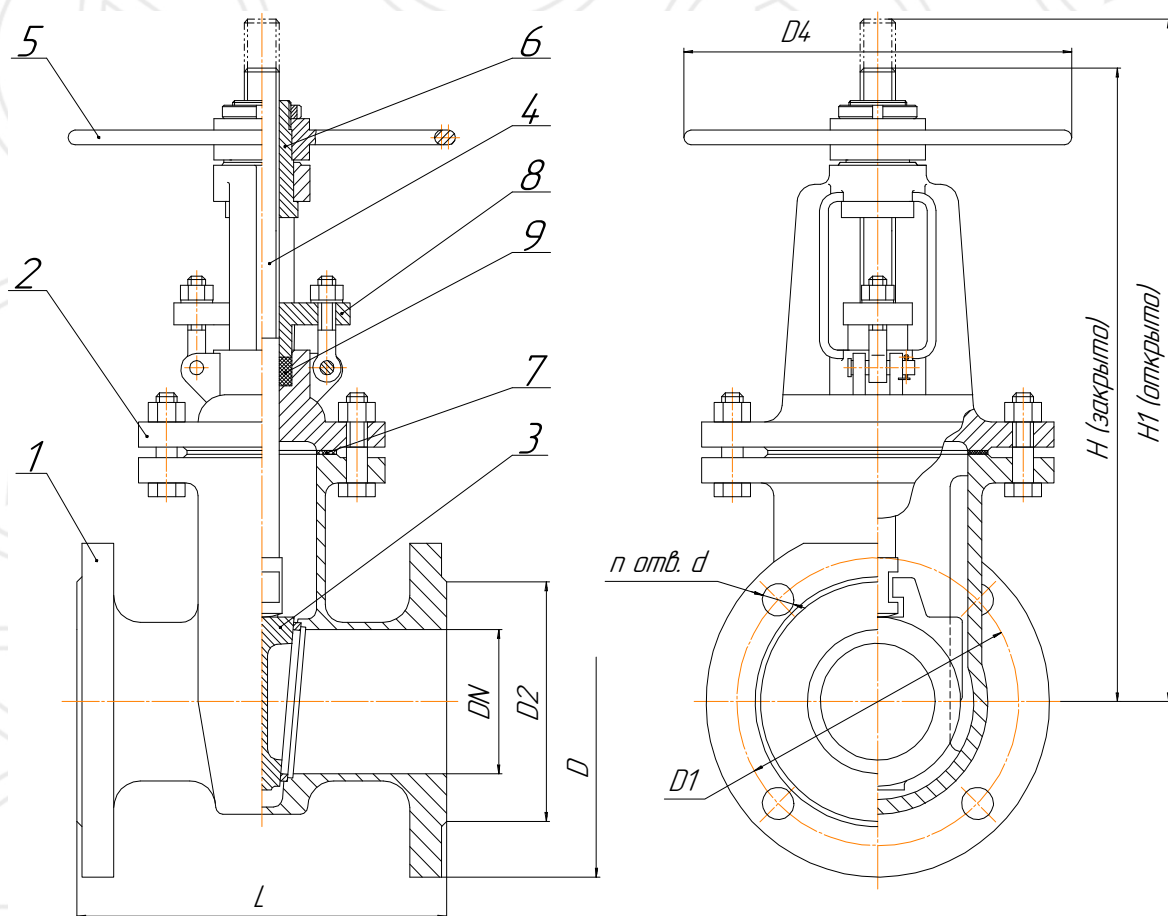
Рисунок 1 Задвижка с выдвижным шпинделем
