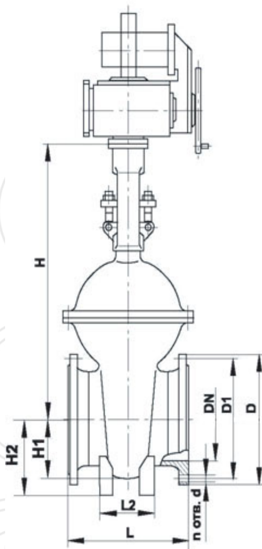
Рисунок 4. Задвижка с не выдвижным шпинделем
