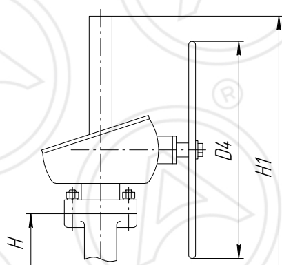
Рисунок 2. Исполнение с редуктором
