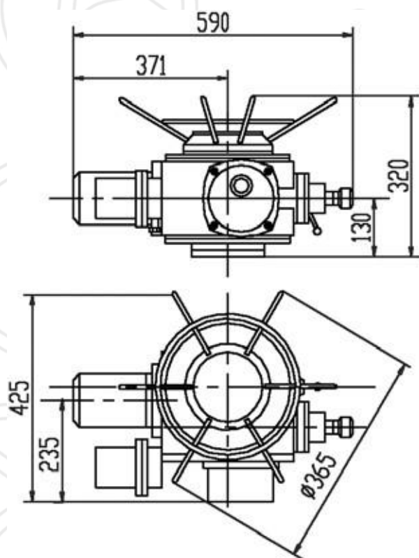
Рис. 8. Внешний вид МЭП-СА3-70, МЭП-СА3-100, МЭП-СА3-150, МЭП-СА3-200, МЭП-СА3-300
