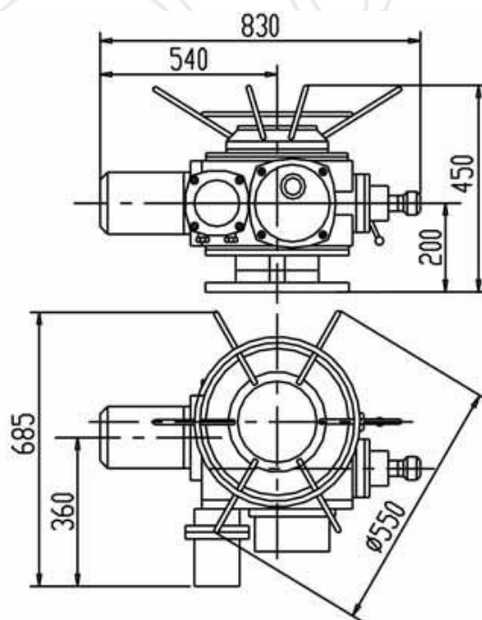
Рис. 10. Внешний вид МЭП-СА3-900, МЭП-СА3-1200
