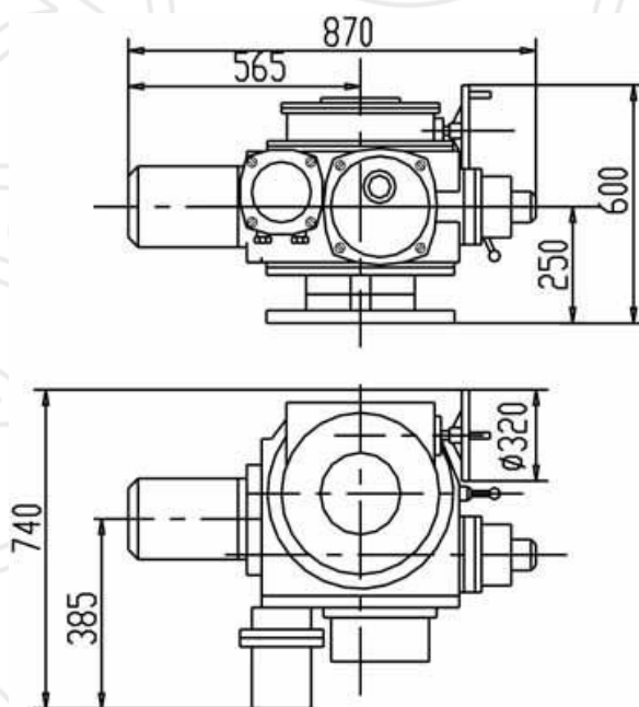
Рис. 11. Внешний вид МЭП-СА3-1800, МЭП-СА3-2500
