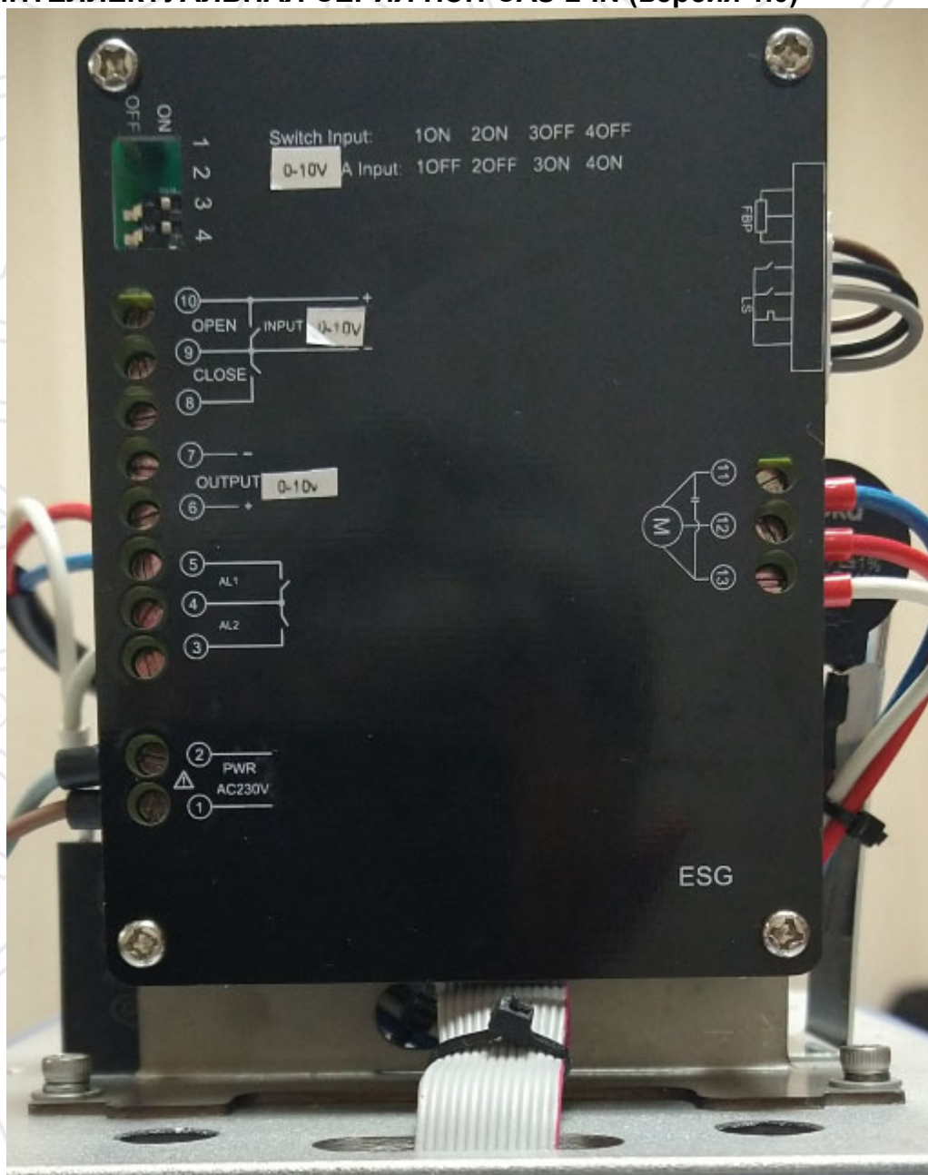
Рис. 13. Клеммы приводов ИНТЕЛЛЕКТУАЛЬНОЙ СЕРИИ (версия 1.0) на усилия 4кН ... 25кН
