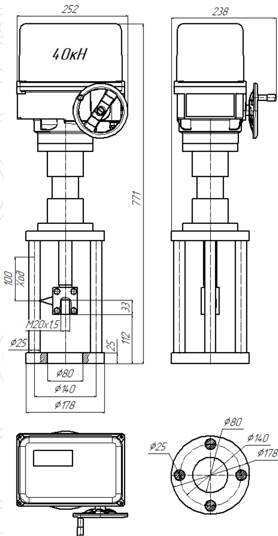
Рис.5 ПЭП-СА3-2-(IN)-40000-100/60-У2-230АС-IP67-0/16
