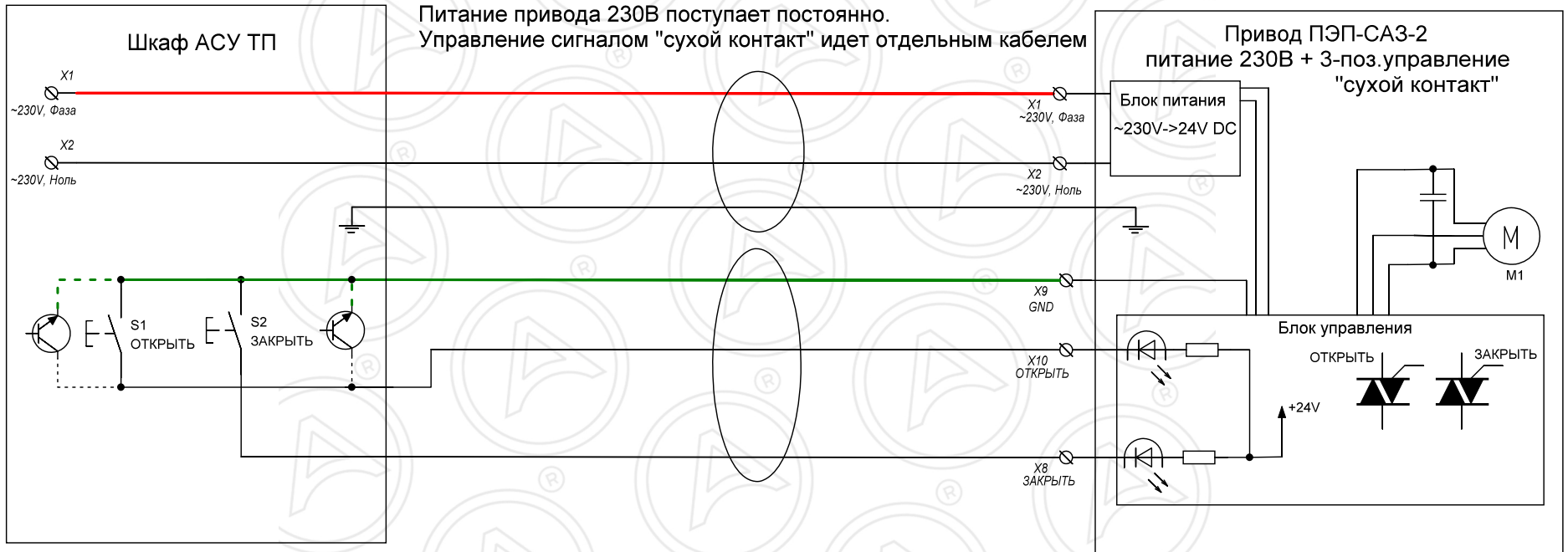
СХЕМА ЗАМЕНЫ КЛАССИЧЕСКОГО 3-ПОЗИЦИОННОГО ПРИВОДА на ПЭП-СА3-2 в режиме трехпозиционного управления
