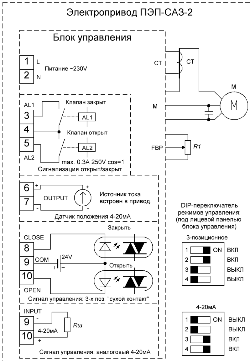
Схема электрического подключения ПЭП-СА3-2
