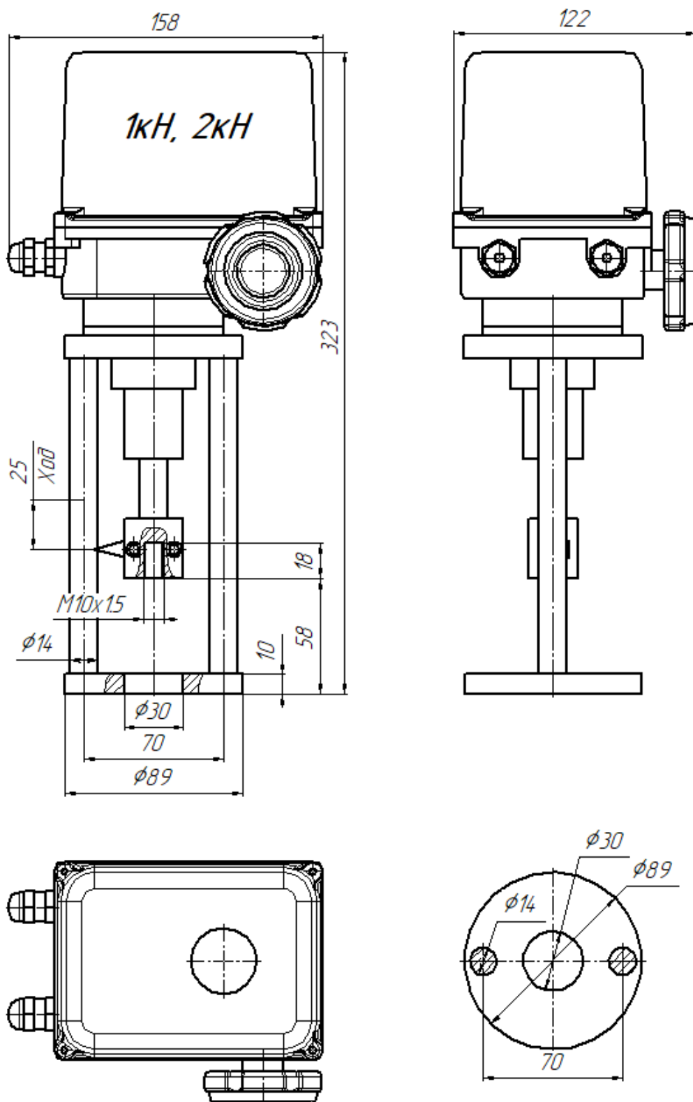
Рис.1 ПЭП-СА3-2-(IN)-1000-25/30-У2-230АС-IP67-0/12, ПЭП-СА3-2-(IN)-2000-25/30-У2-230АС-IP67-0/12
