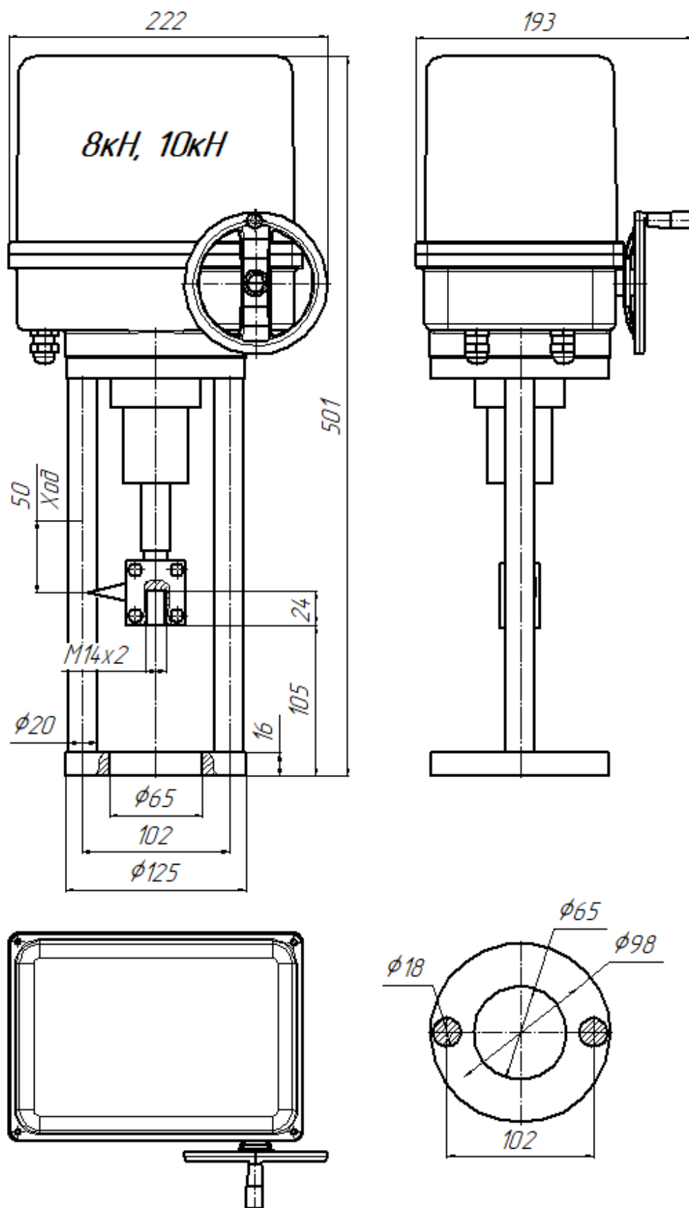
Рис.3 ПЭП-СА3-2-(IN)-8000-50/40-У2-230АС-IP67-0/14, ПЭП-СА3-2-(IN)-10000-50/40-У2-230АС-IP67-0/14
