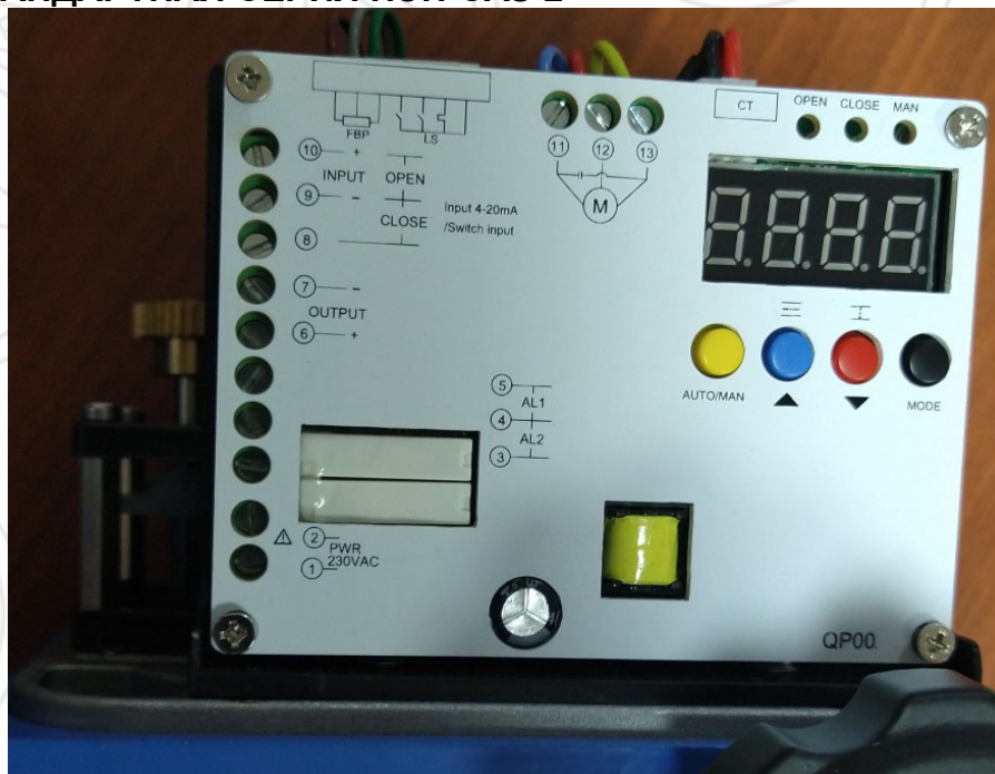
Рис. 11. Клеммы приводов СТАНДАРТНОЙ СЕРИИ на усилия 1кН и 2кН
