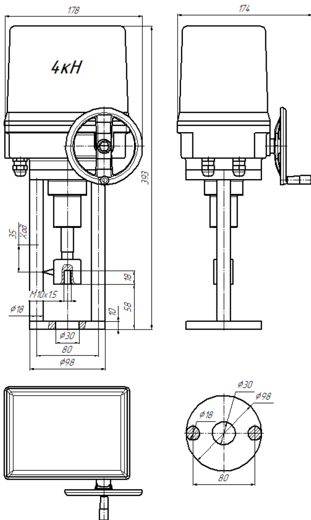
Рис.2 ПЭП-СА3-2-4000-35/35-У2-230АС-IP67-0/13
