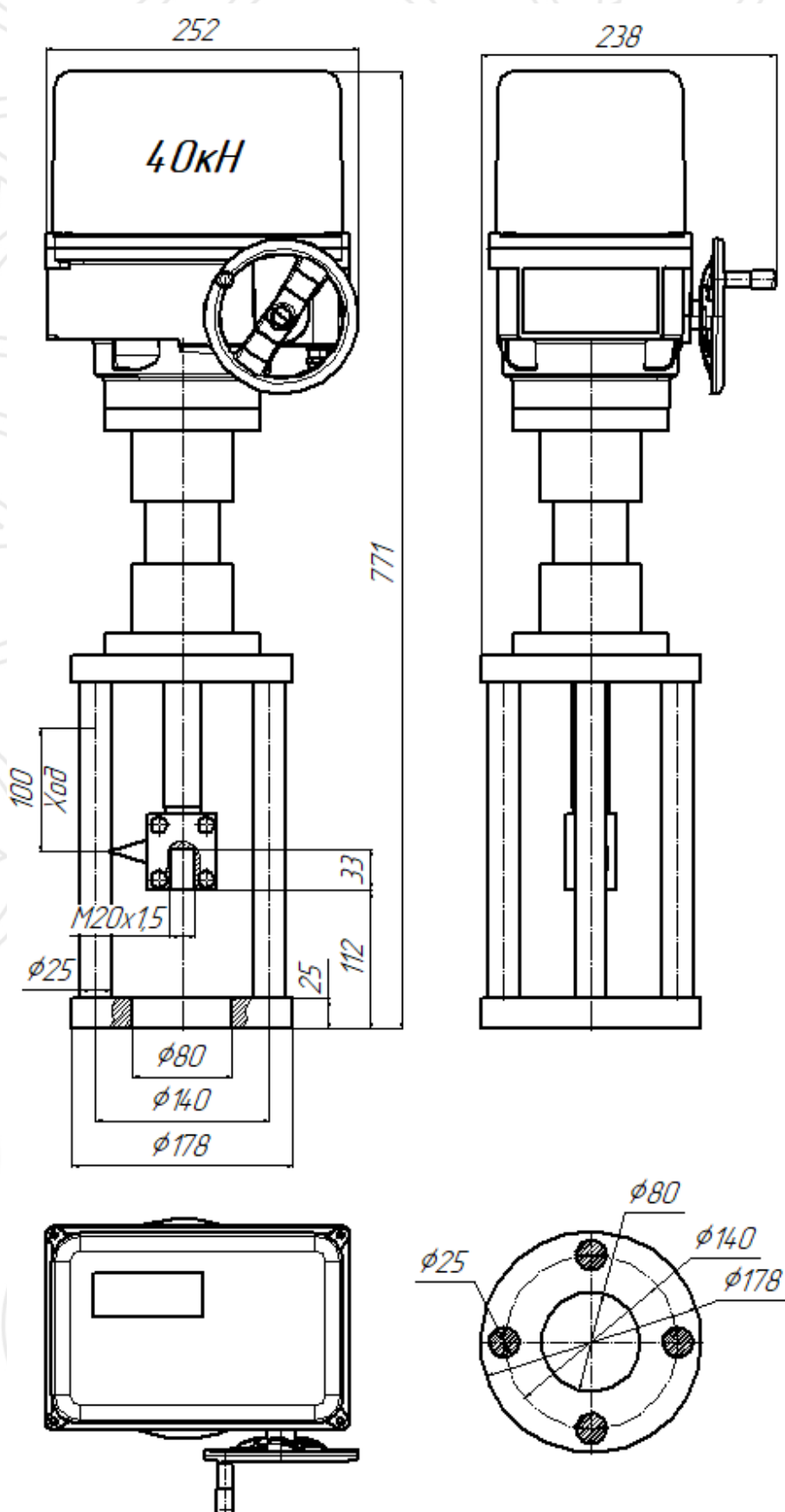
Рис.5 ПЭП-САЗ-2-40000-100/60-У2-230АС-IP67-0/16
