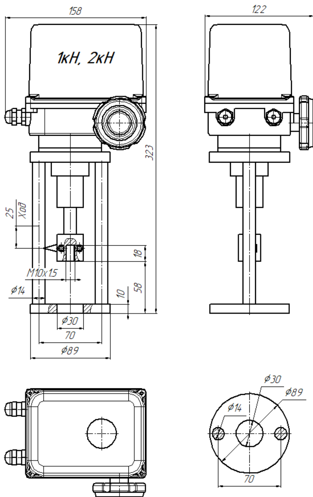
Рис.1 ПЭП-СА3-2-1000-25/30-У2-230АС-IP67-0/12, ПЭП-СА3-2-2000-25/30-У2-230АС-IP67-0/12
