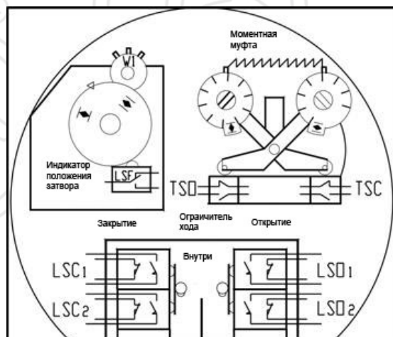
Рис. 7. Схема расположения электрических элементов
