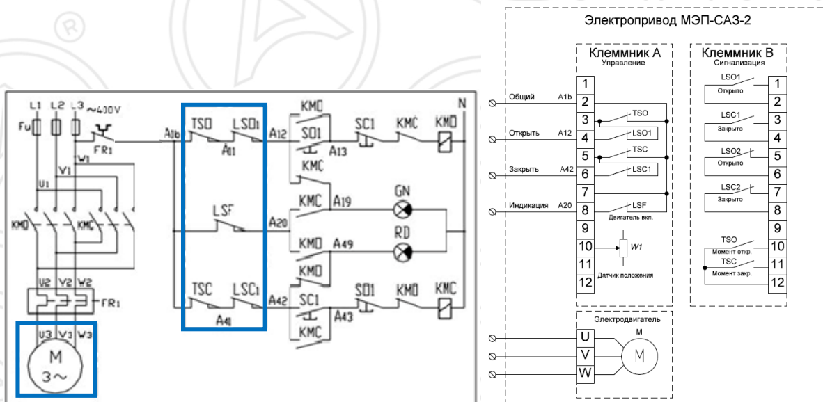
Рис. 6. – Электрическая схема управления
